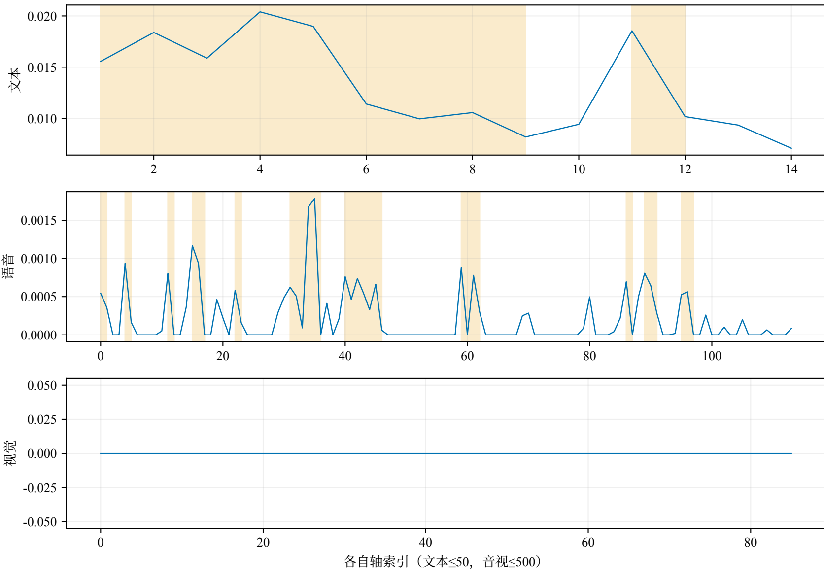
样本 11 正向 Grad×Input（支持当前预测）
