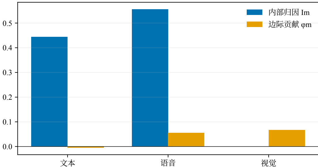
样本 13 三模态作用差异
