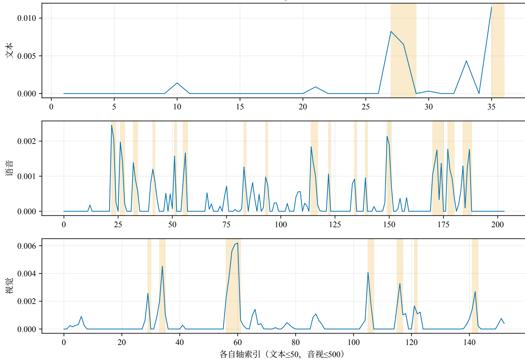
样本 14 正向 Grad×Input（支持当前预测）
