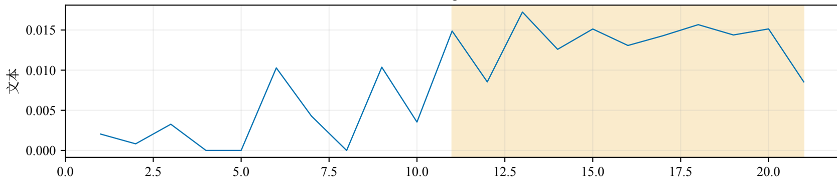
样本 15 正向 Grad×Input（支持当前预测）
