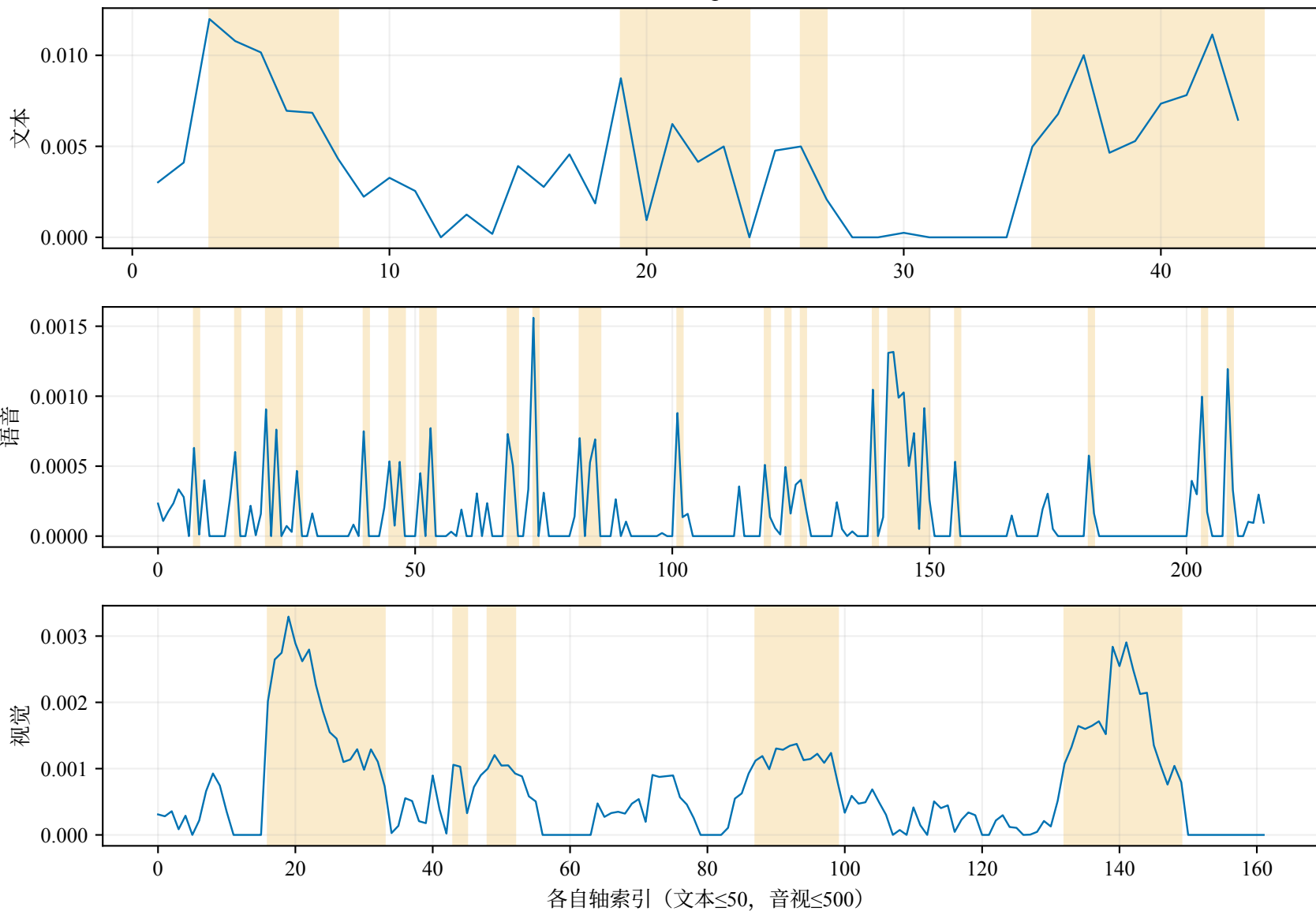
样本 20 正向 Grad×Input（支持当前预测）
