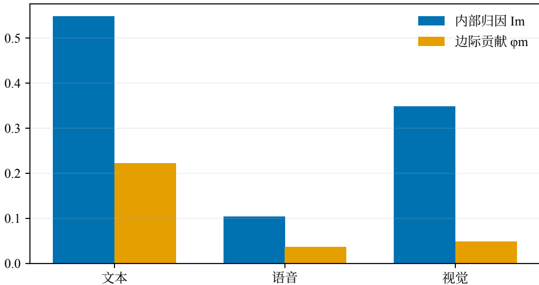
样本 20 三模态作用差异
