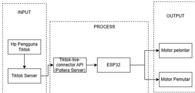
Gambar 6. Blok Diagram Sistem.
