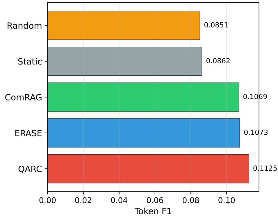
Token F1
