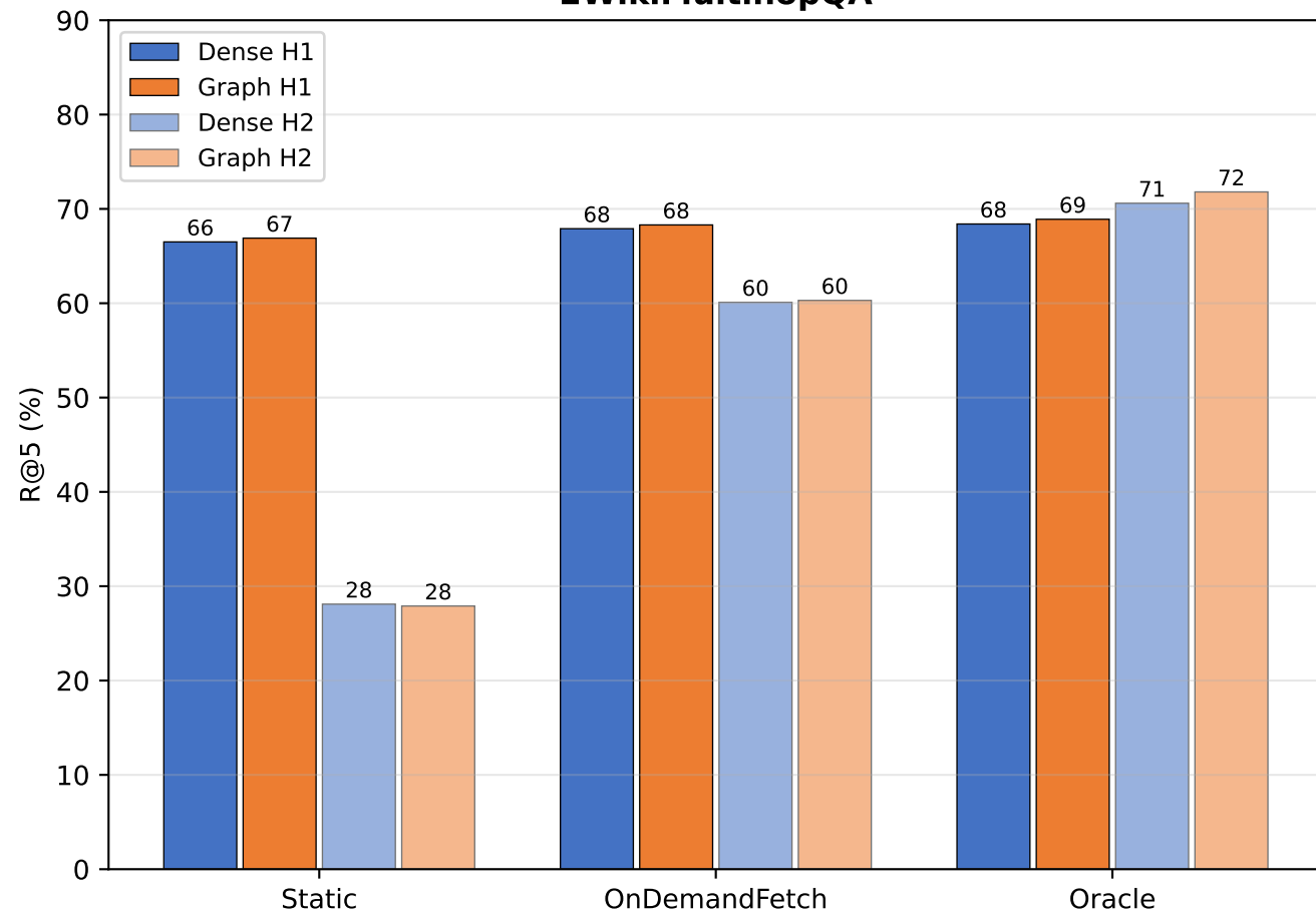
2WikiMultihopQA
