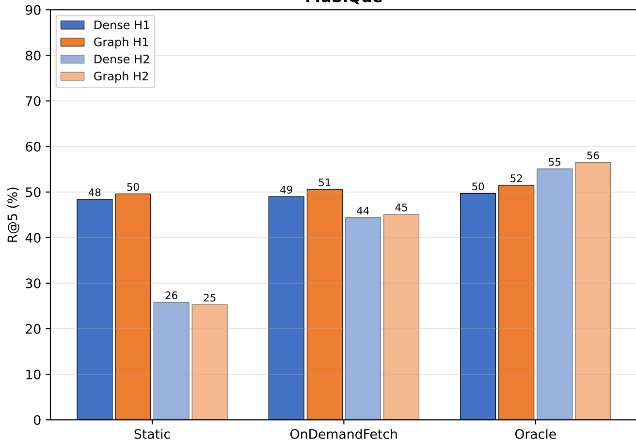
MuSiQue
