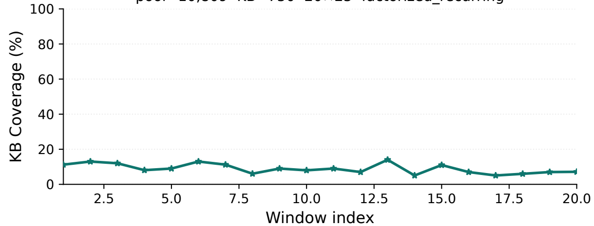
2WikiMultihopQA
