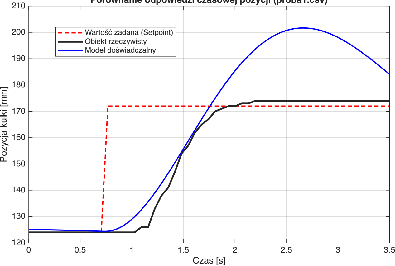
Porównanie odpowiedzi czasowej pozycji (proba1.csv)
