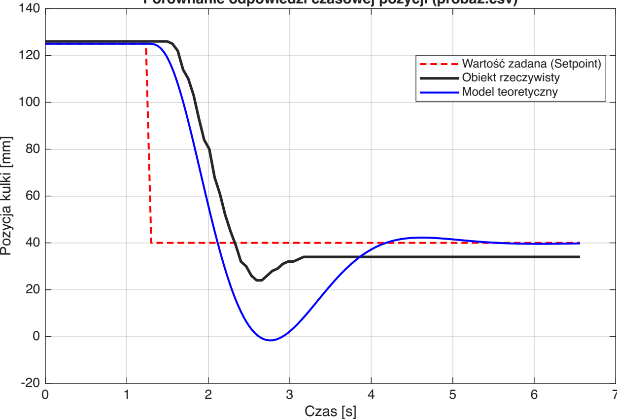
Porównanie odpowiedzi czasowej pozycji (proba2.csv)
