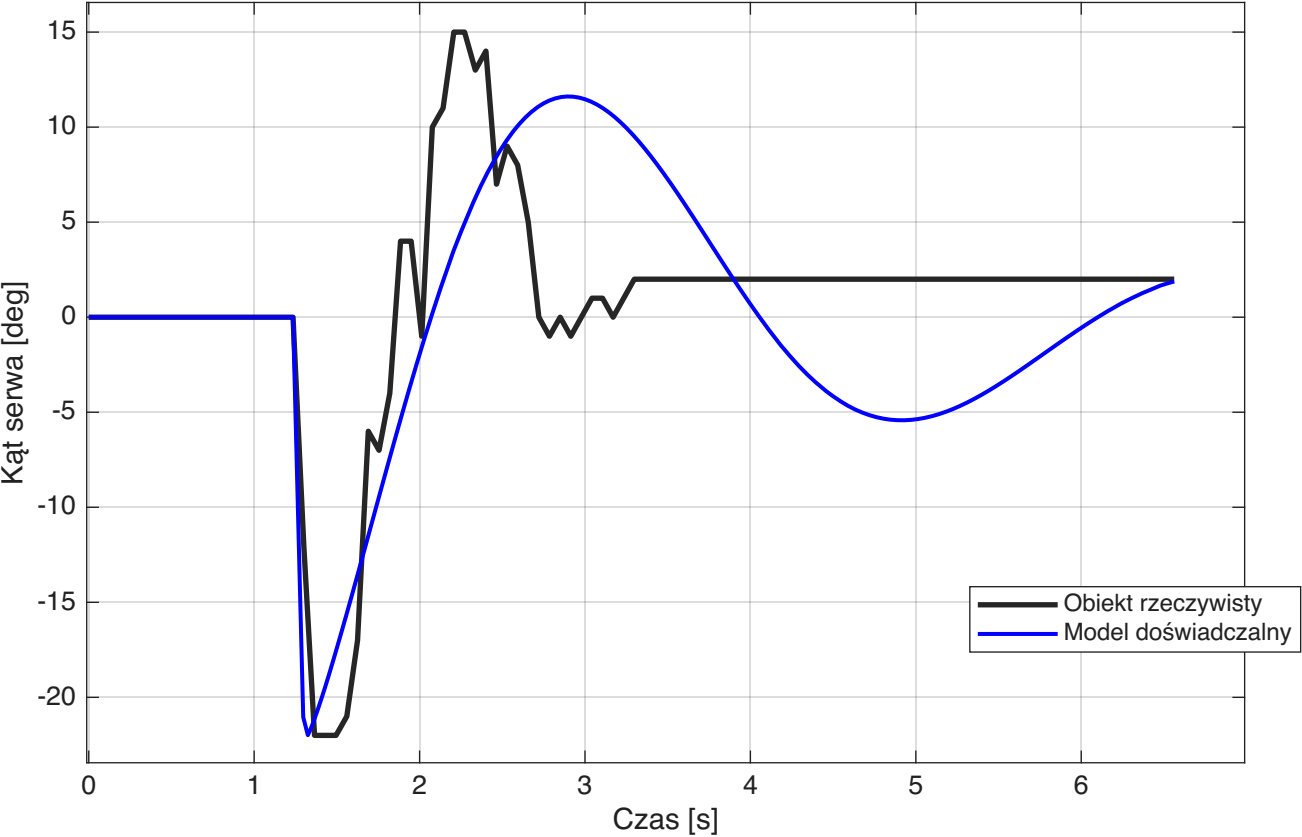
Porównanie sygnału sterującego (proba2.csv)
