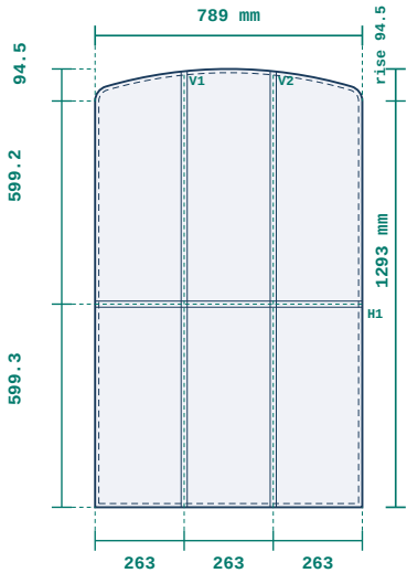
2 · TC-BARS — ARCHED LEAF GLASS double 4x16x4 · toughened · Standard · Argon · clear · spacer: silver (warm edge) · bars: 1H x 2V astragal · arched · R 44.5/1294.5 · rise 94.5 · springing 1198.5
