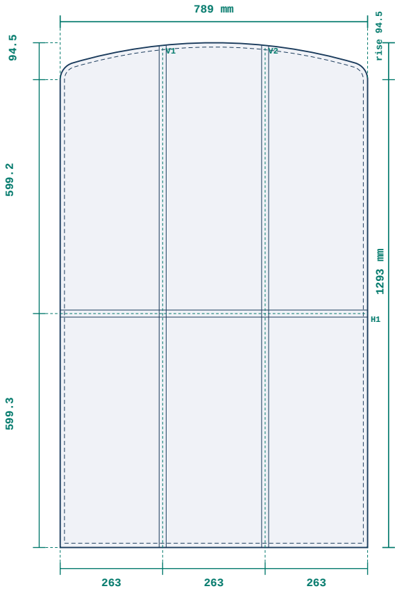
2 · TC-BARS — ARCHED LEAF GLASS double 4x16x4 · toughened · Standard · Argon · clear · spacer: silver (warm edge) · bars: 1H x 2V astragal · arched · R 44.5/1294.5 · rise 94.5 · springing 1198.5
