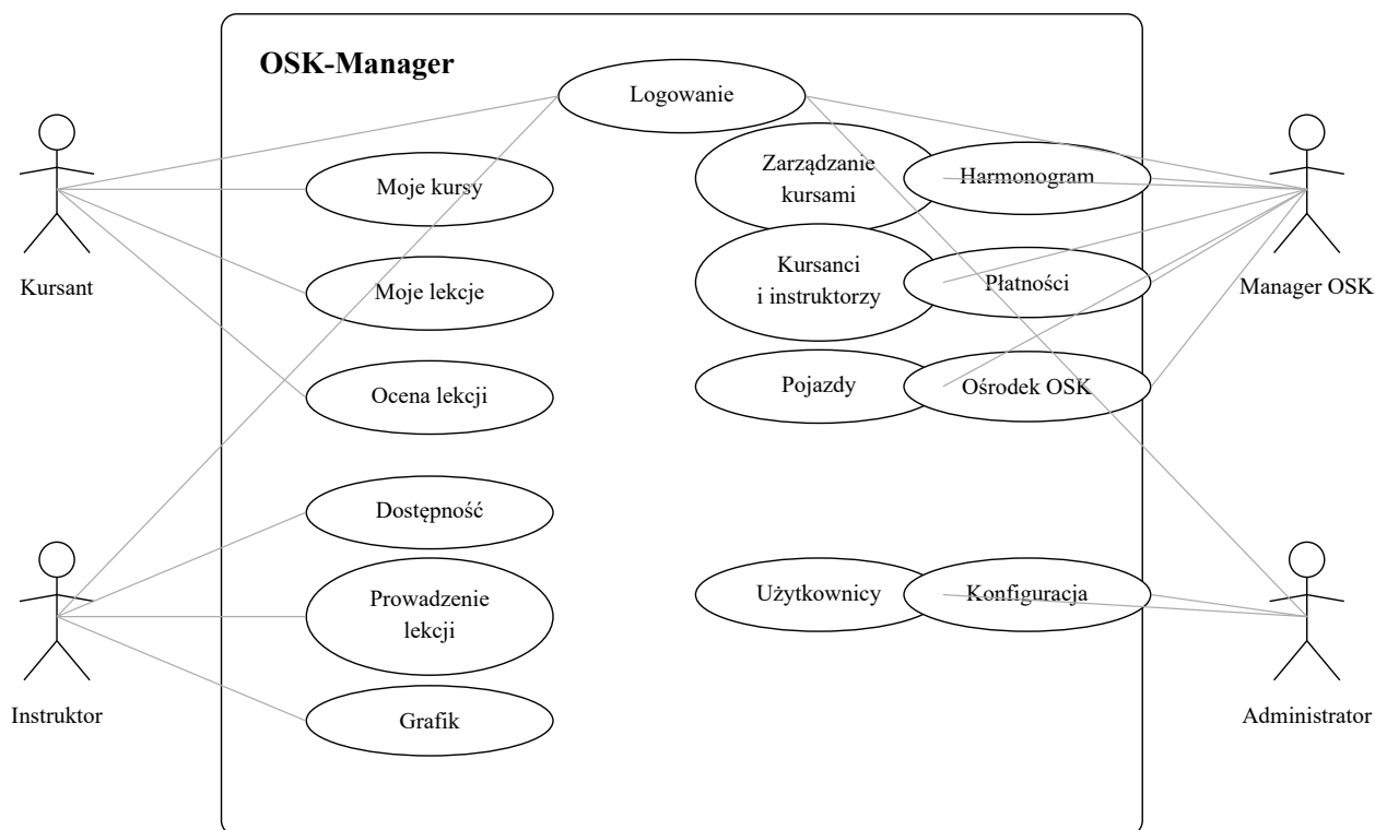
Rys. 3.1. Diagram przypadków użycia systemu OSK-Manager
