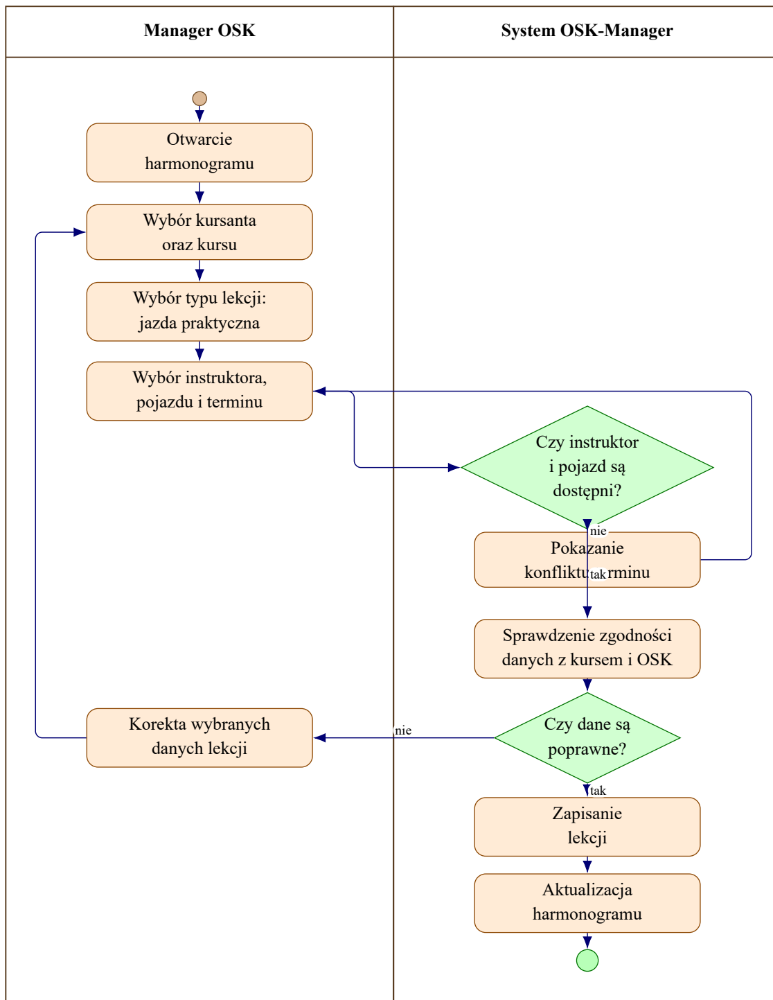
Rys. 3.2. Diagram aktywności procesu planowania lekcji praktycznej
