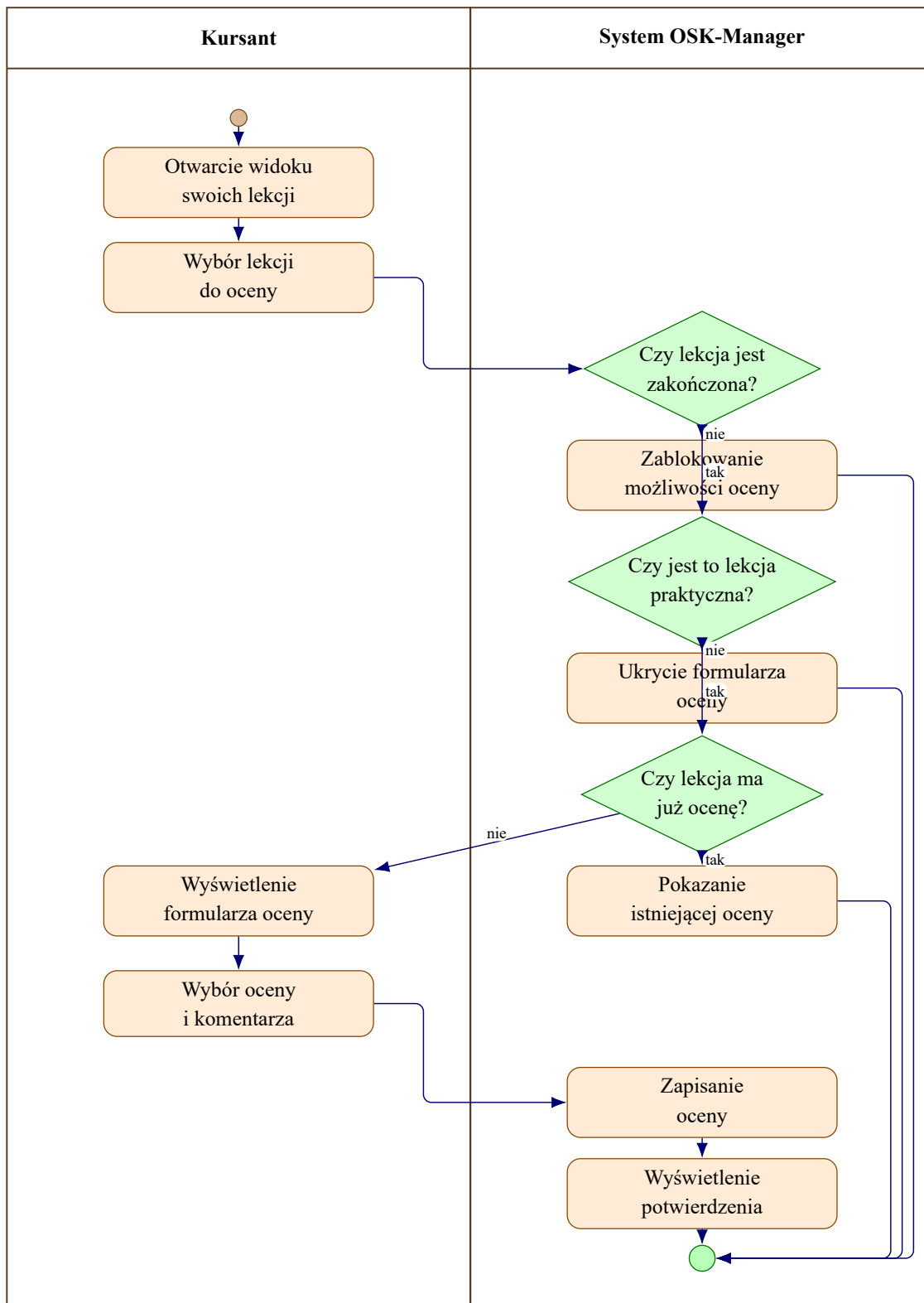
Rys. 3.3. Diagram aktywności procesu oceny zakończonej lekcji
