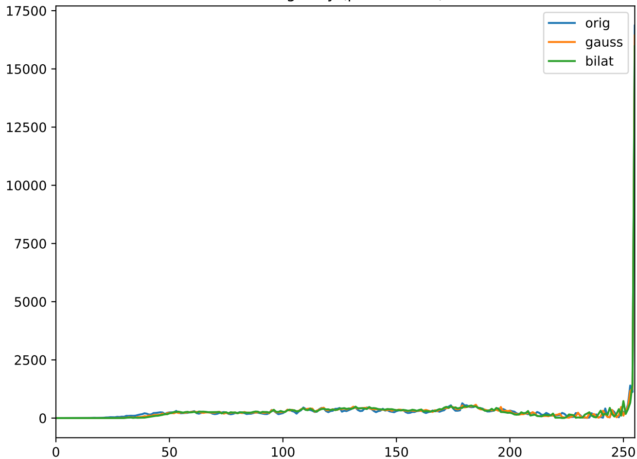
Histogramy (porównanie)
