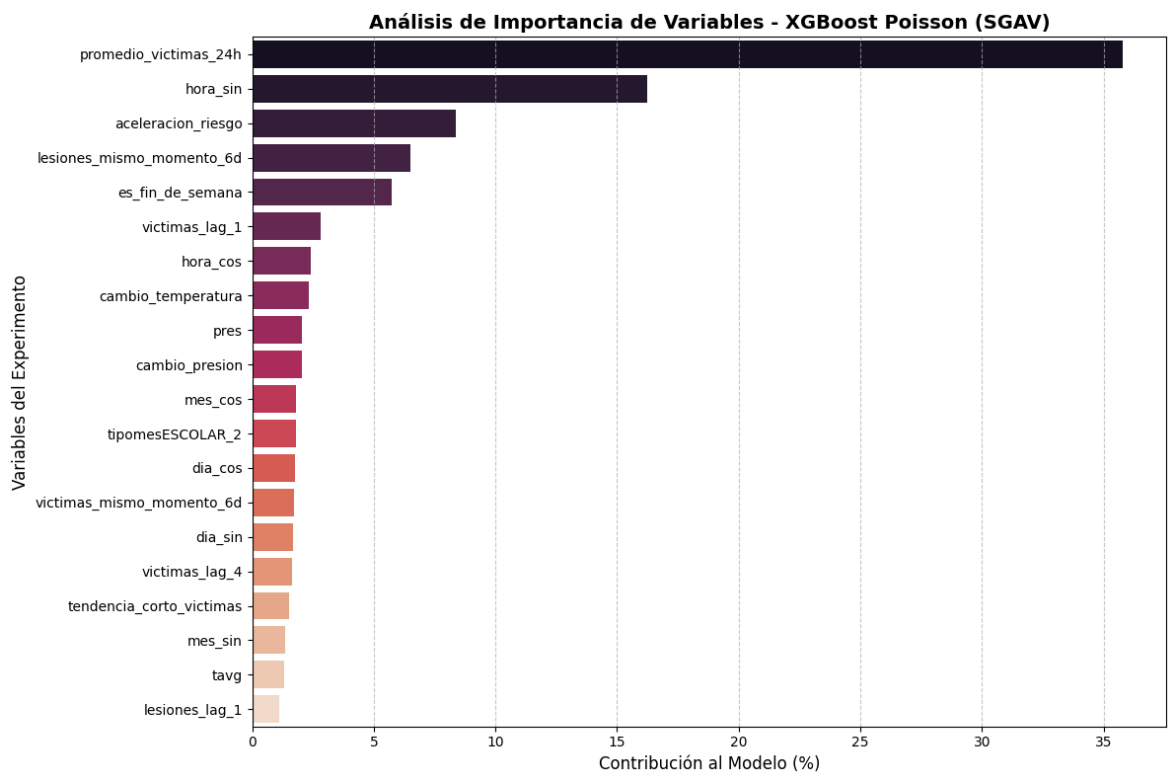
Figura 3.13: Contribución de cada variable a la capacidad de predicción del modelo Nota. Elaboración propia, según la salida del modelo entrenado.
