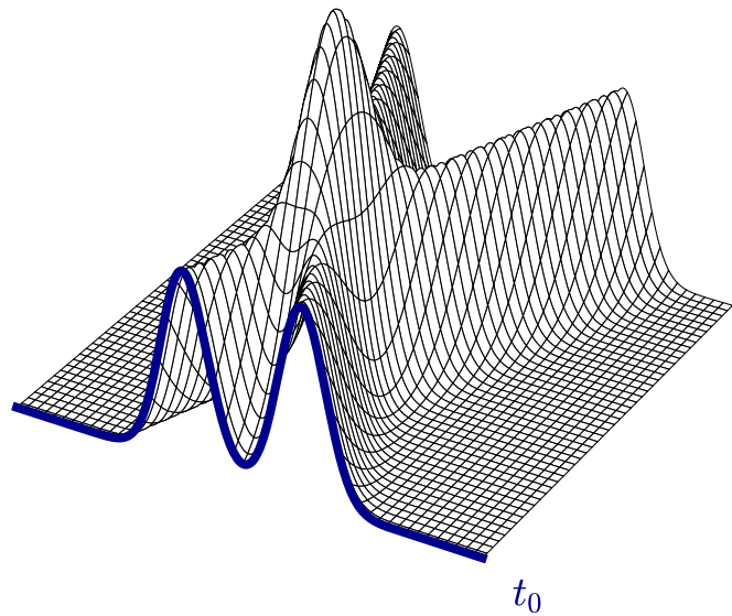
Interferenza costruttiva
