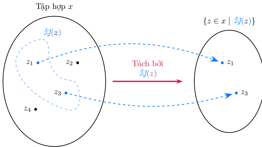
Hình 1.6: Minh họa tiên đề tách (các phần tử của x thỏa mãn tính chất \dot{\mathcal{A}}(z) được tách ra).
