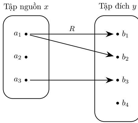
Hình 1.8: Minh họa quan hệ R \subseteq x \times y với các cặp (a_1; b_1), (a_1; b_2), (a_3; b_3) thuộc R .
