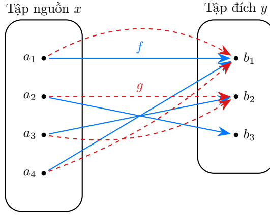
Hình 1.11: Minh họa ánh xạ f là toàn ánh và ánh xạ g không phải là toàn ánh.
