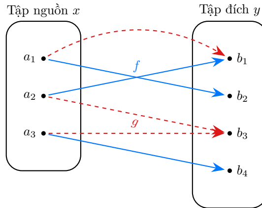
Hình 1.10: Minh họa ánh xạ f là đơn ánh và ánh xạ g không phải là đơn ánh.
