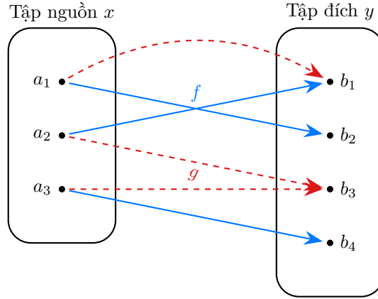
Hình 1.3: Minh họa ánh xạ f là đơn ánh và ánh xạ g không phải là đơn ánh.
