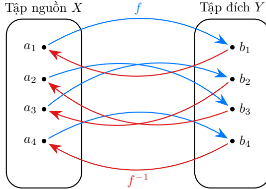
Hình 1.5: Minh họa ánh xạ f là ánh xạ song ánh.
