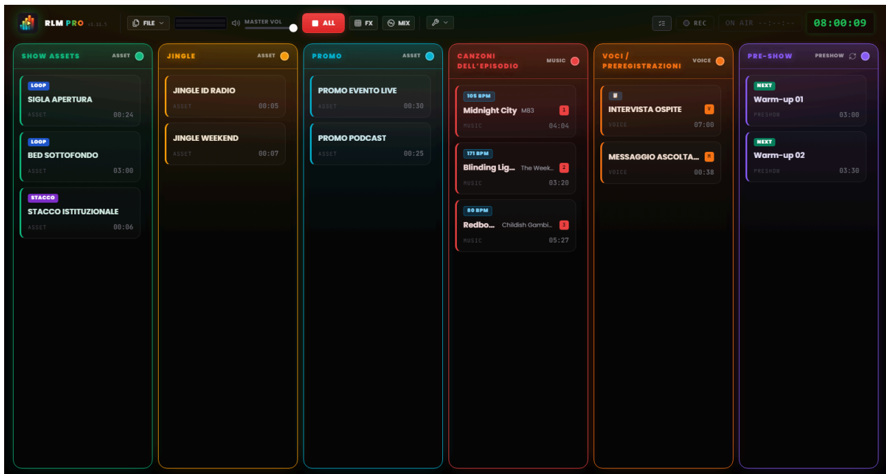
Figura 3.2 — L'interfaccia di lavoro: la griglia a sei colonne con le card audio.
