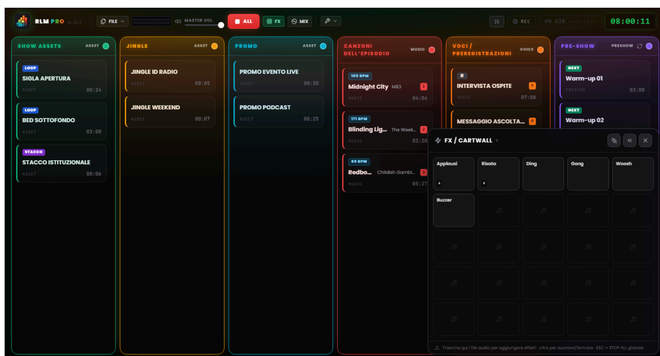
Figura 7.1 — Il pad FX: la jingle machine 5×5 degli effetti sonori, con lancio a sovrapposizione.
