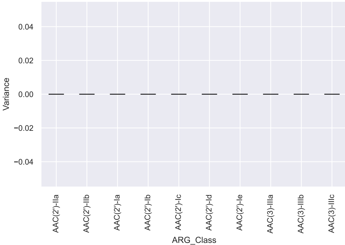
Top Variable ARGs
