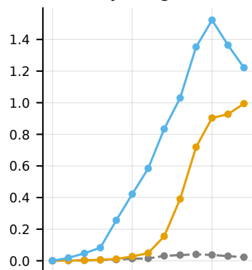
Tiny ImageNet
