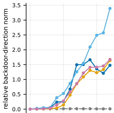
GTSRB
