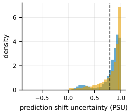
CIFAR-10, WaNet 10% (AUROC 0.459)
