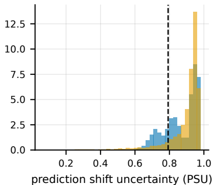
CIFAR-10, SIG 10% (AUROC 0.418)
