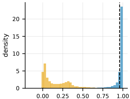
CIFAR-10, WaNet 10% (AUROC 0.459)
