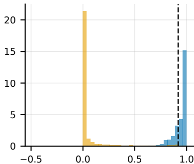
CIFAR-10, SIG 10% (AUROC 0.418)
