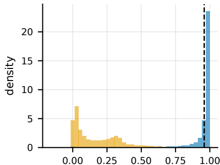
GTSRB, TaCT 1% (AUROC 0.266)
