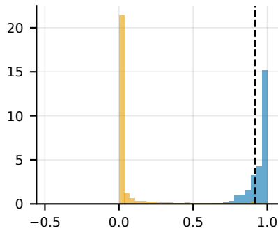
CIFAR-10, WaNet 10% (AUROC 0.459)
