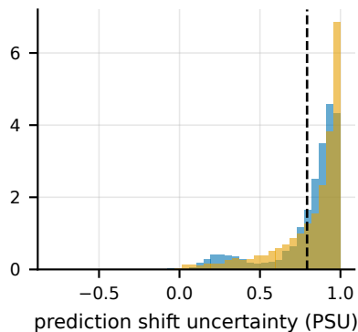
CIFAR-10, WaNet 10% (AUROC 0.459)
