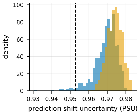
GTSRB, TaCT 1% (AUROC 0.266)
