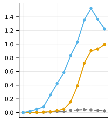
Tiny ImageNet
