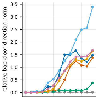
GTSRB
