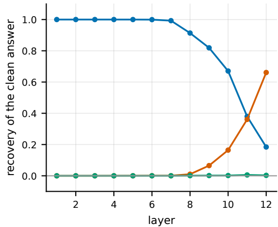
BadNets (n=12)
