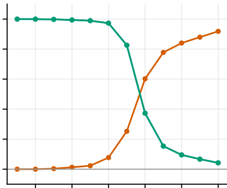
Blend (n=12)
