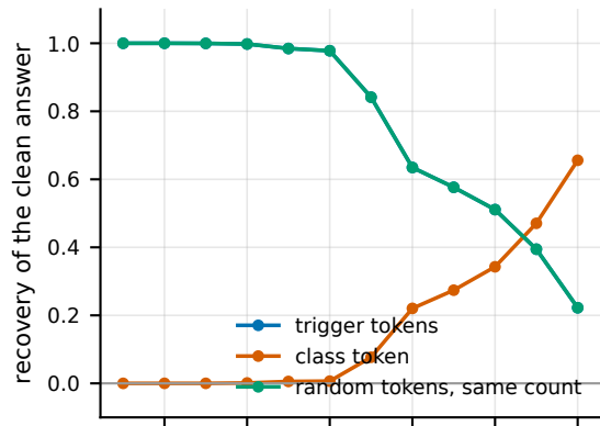
BadNets (n=12)
