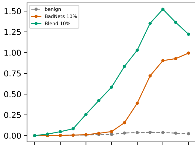
Tiny ImageNet
