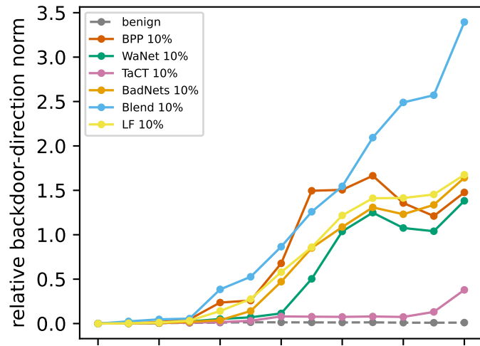
GTSRB
