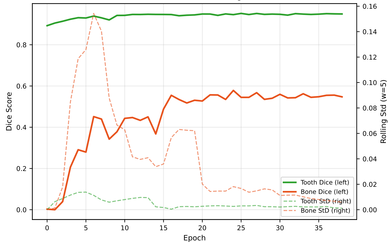
A. Validation Dice + Rolling Std
