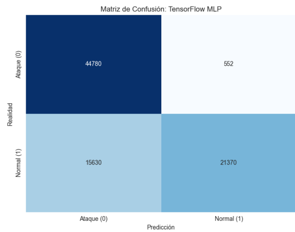
Figura 26. MC - MLP
