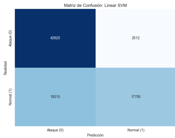
Figura 25. MC - SVM
