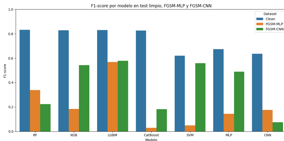
Figura 61. F1-FGSM-UNSW-NB15
