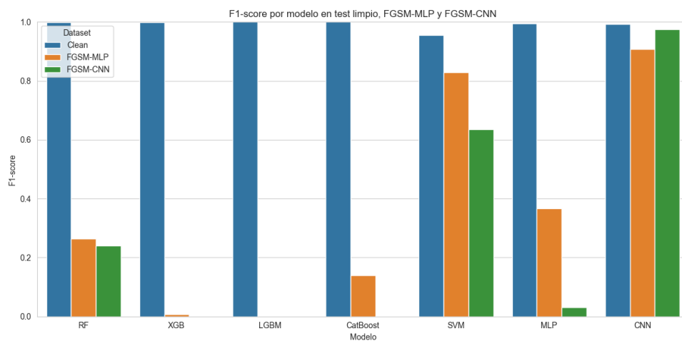
Figura 67. F1-FGSM-IOT-23
