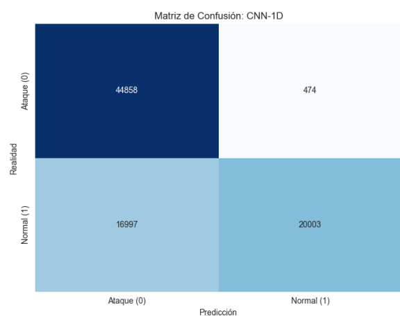
Figura 27. MC - CNN
