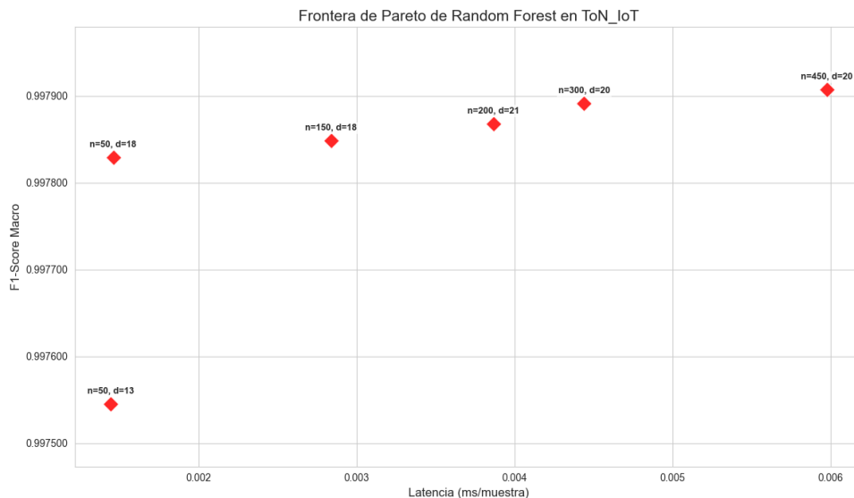
Figura 43. Frontera de Pareto - Random Forest (ToN-IoT)
