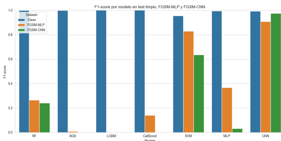
Figura 2.55. F1-FGSM-IOT-23
