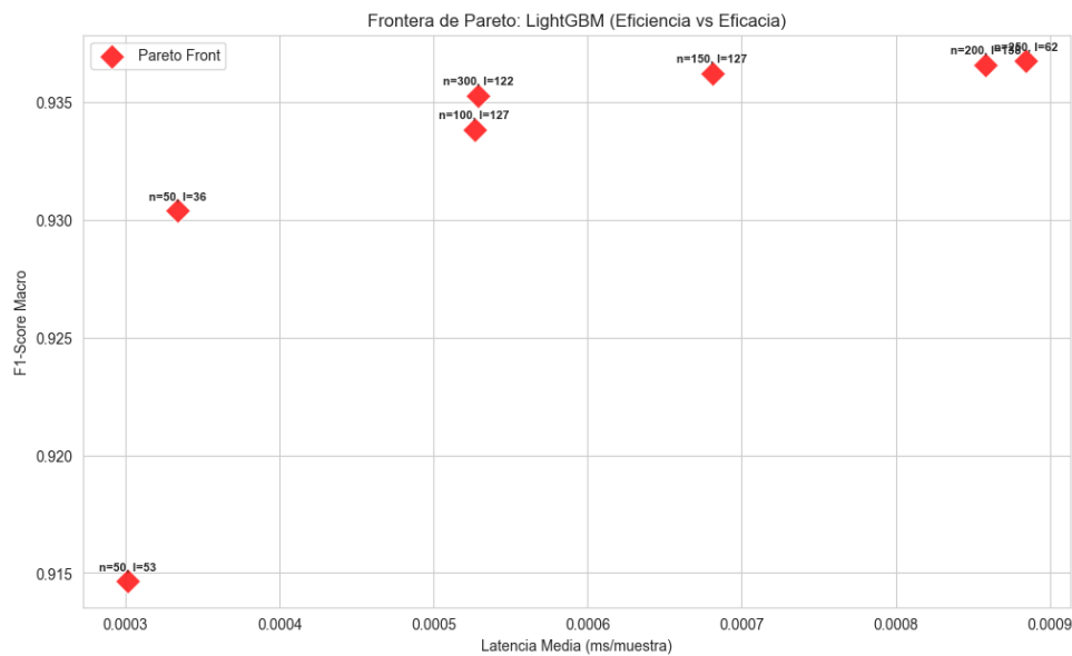
Figura 14. Frontera de Pareto - LightGBM
