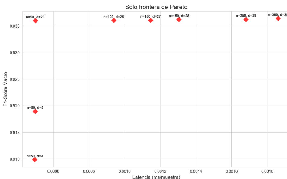
Figura 12. Frontera de Pareto - Random Forest
