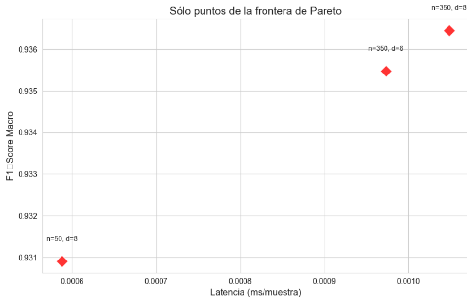
Figura 13. Frontera de Pareto - XGBoost
