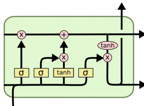
Figura 6. Esquema representativo de una unidad LSTM con sus compuertas internas.
