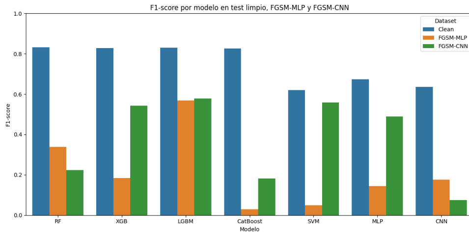
Figura 2.49. F1-FGSM-UNSW-NB15
