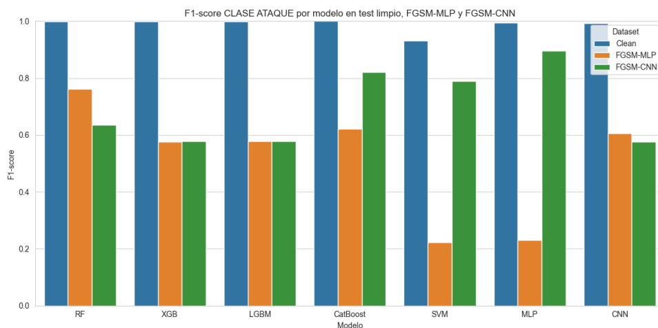
Figura 2.55. F1-FGSM-IOT-23
