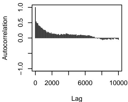
traitX80.56.8:traitX483.76.1.specie
