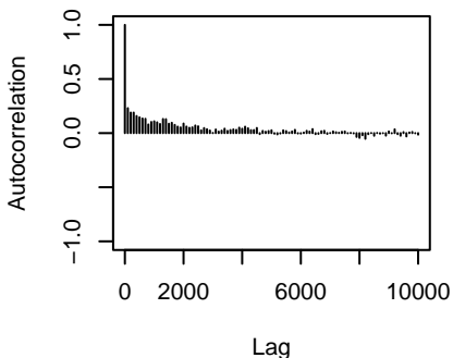
traitX79.92.5:traitX483.76.1.units
