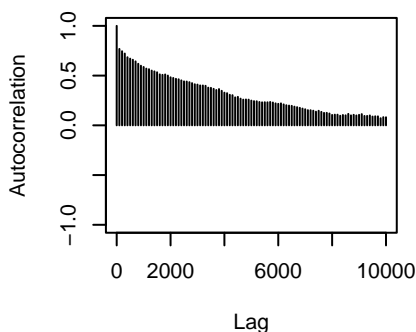
traitX87.44.5:traitX138.86.3.specie
