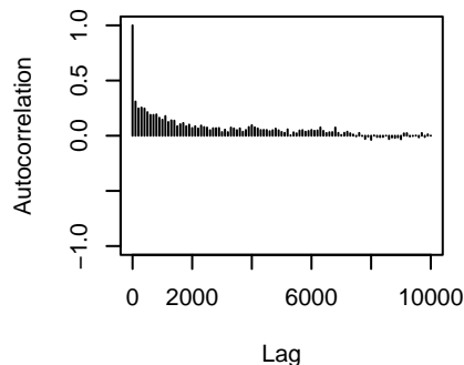
traitX483.76.1:traitX87.44.5.units
