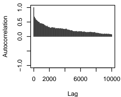
traitX123.35.3:traitX79.92.5.specie
