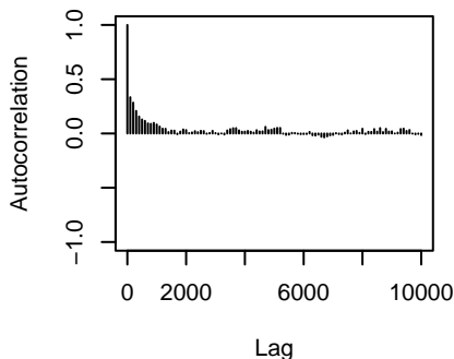
traitX127.91.3:traitX562.74.3.unit
