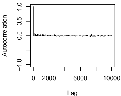
traitX98.55.5:traitX562.74.3.units
