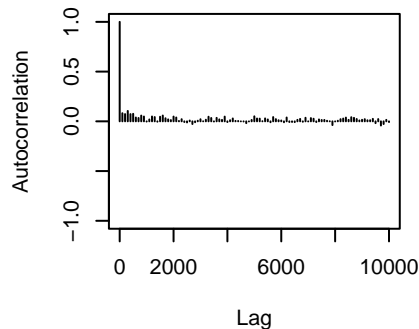
traitX562.74.3:traitX79.92.5.units
