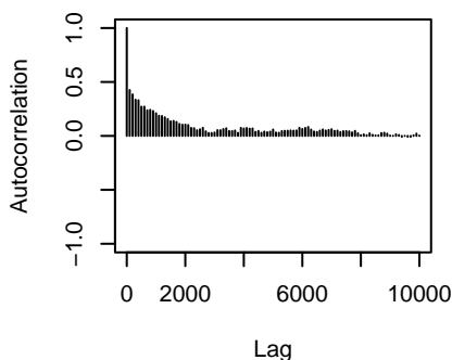
traitX127.91.3:traitX98.55.5.specie
