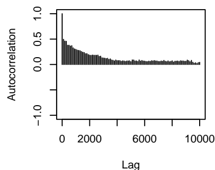
traitX138.86.3:traitX562.74.3.specie
