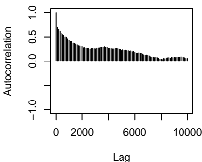
traitX483.76.1:traitX483.76.1.specie
