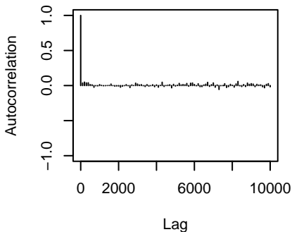
traitX80.56.8:traitX98.55.5.units
