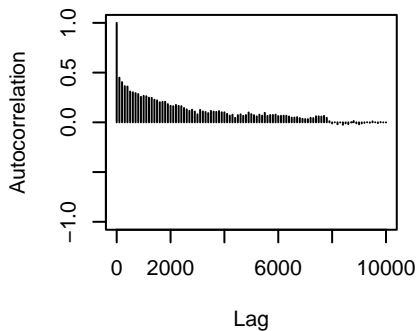
traitX87.44.5:traitX127.91.3.specie
