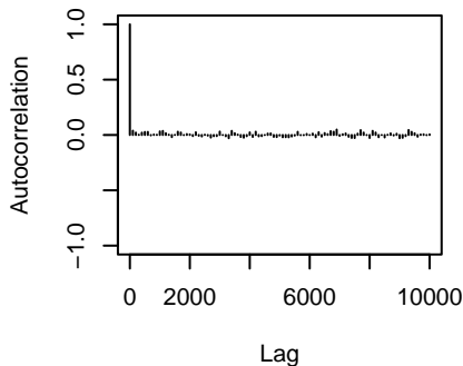
traitX123.35.3:traitX562.74.3.unit
