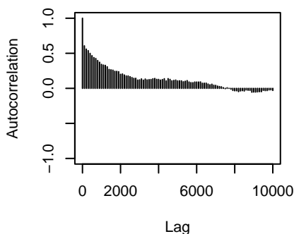
traitX87.44.5:traitX80.56.8.specie
