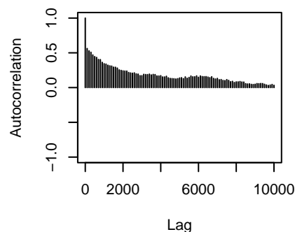
traitX483.76.1:traitX98.55.5.specie
