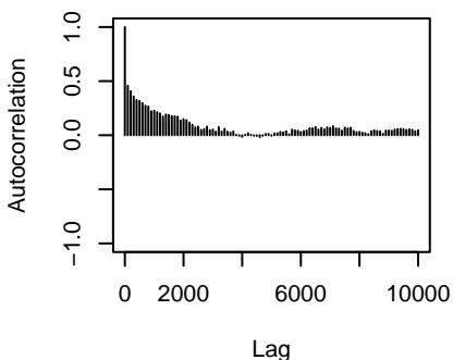
traitX79.92.5:traitX127.91.3.units
