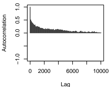
traitX79.92.5:traitX562.74.3.specie
