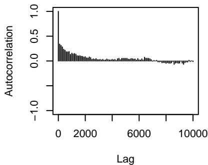
traitX87.44.5:traitX80.56.8.units
