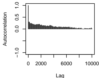
traitX138.86.3:traitX79.92.5.units
