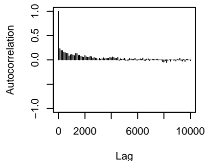
traitX483.76.1:traitX79.92.5.units
