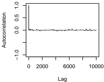
traitX80.56.8:traitX80.56.8.units
