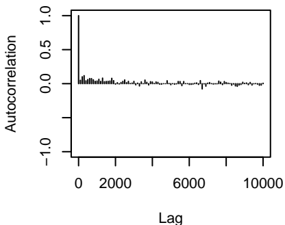
traitX98.55.5:traitX138.86.3.units
