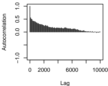
traitX562.74.3:traitX483.76.1.specie
