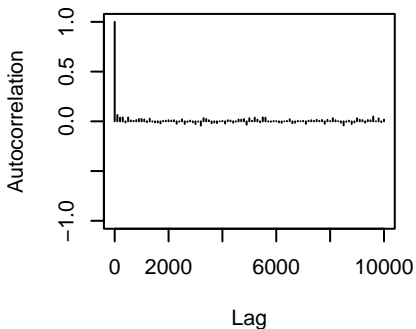
traitX80.56.8:traitX138.86.3.units
