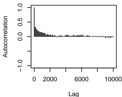
traitX87.44.5:traitX98.55.5.specie
