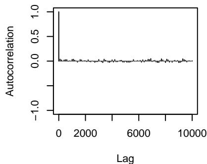
traitX562.74.3:traitX123.35.3.unit
