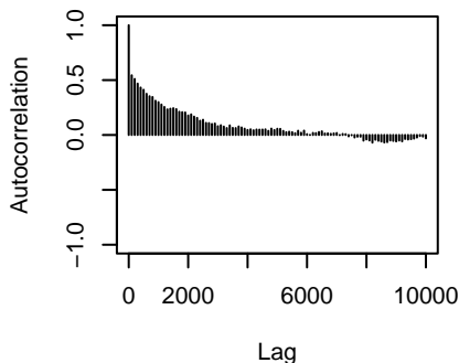
traitX87.44.5:traitX87.44.5.units
