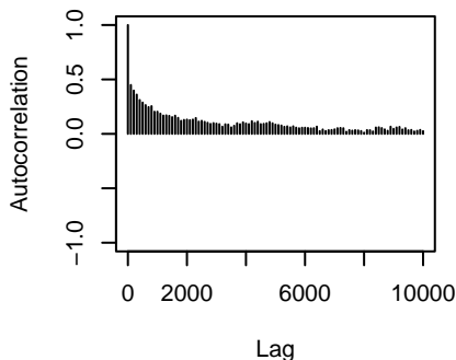
traitX127.91.3:traitX483.76.1.unit
