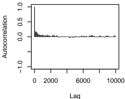
traitX79.92.5:traitX98.55.5.units
