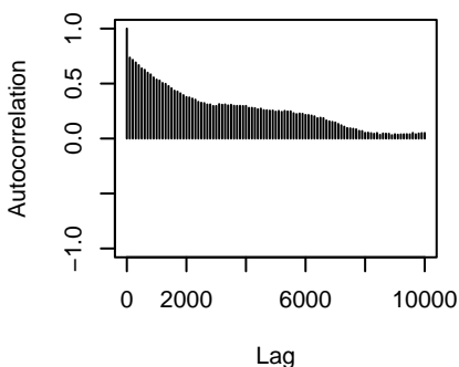
traitX79.92.5:traitX483.76.1.specie
