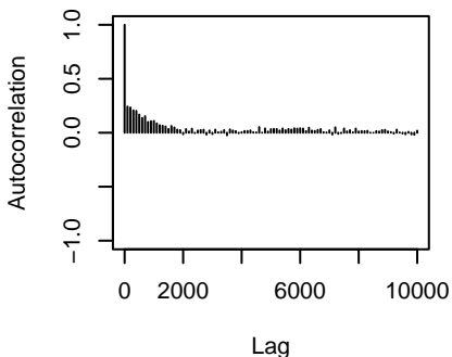
traitX79.92.5:traitX79.92.5.units
