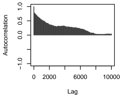
traitX483.76.1:traitX127.91.3.specie
