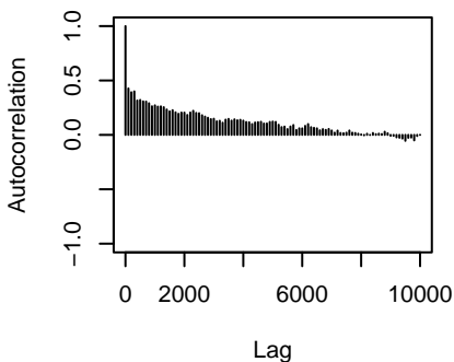
traitX80.56.8:traitX562.74.3.specie
