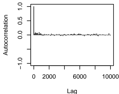
traitX138.86.3:traitX483.76.1.units
