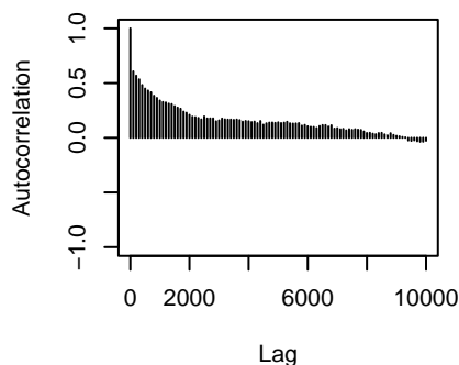
traitX483.76.1:traitX123.35.3.specie
