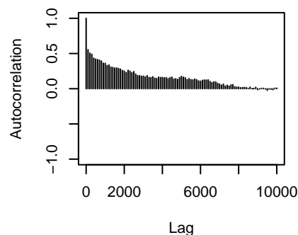
traitX483.76.1:traitX562.74.3.specie
