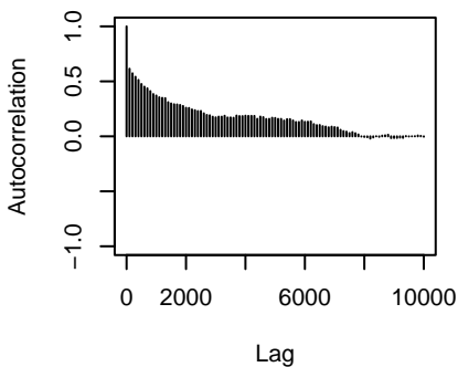
traitX80.56.8:traitX127.91.3.specie
