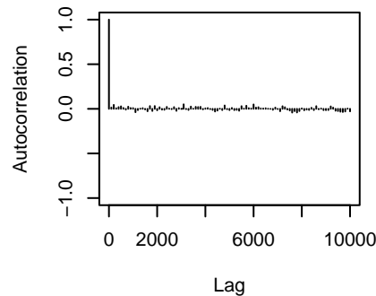
traitX562.74.3:traitX80.56.8.units
