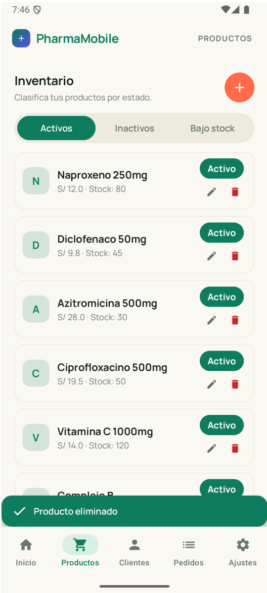
Figura 4. "Producto eliminado" tras el DELETE (204).
