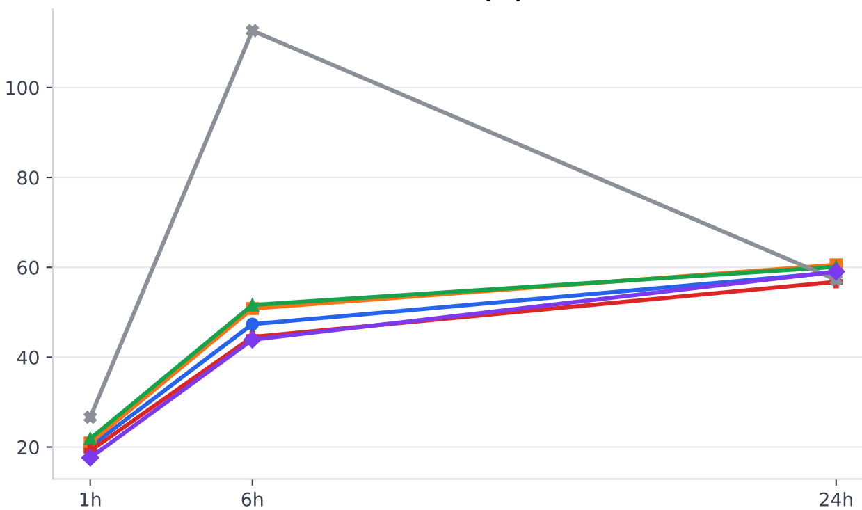
PINAW (80% PI)
