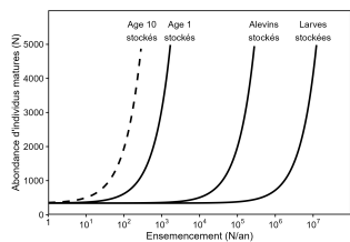
Fig. 3. Résultats de notre analyse. Est représenté : L'effet d'augmenter l'ensemencement de larves, alevins, individus d'âge 1, et individus matures (âge 10) sur l'abondance de chevaliers matures sur 100 ans dans notre scénario mesuré. Lors de l'application aux scénarios nules et menacés, les résultats étaient indistinguables de ceux présentés.
