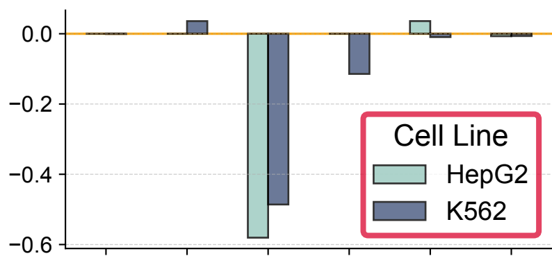
Avg. SHAP
