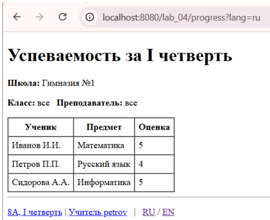
Рисунок 1 – Результат работы сервлета
