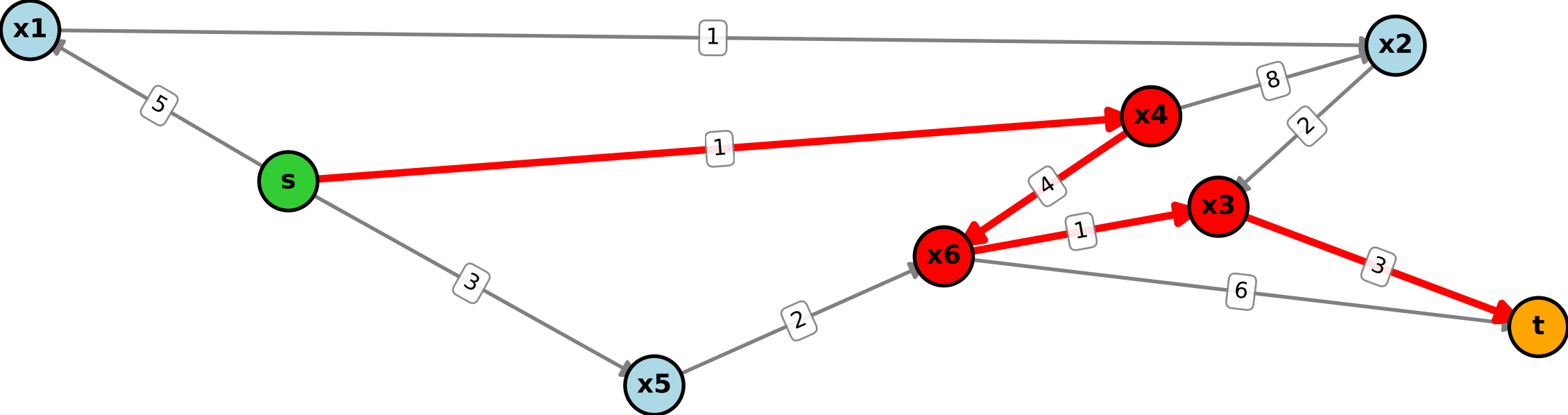
Орграф с кратчайшим путем от 's' к 't'
