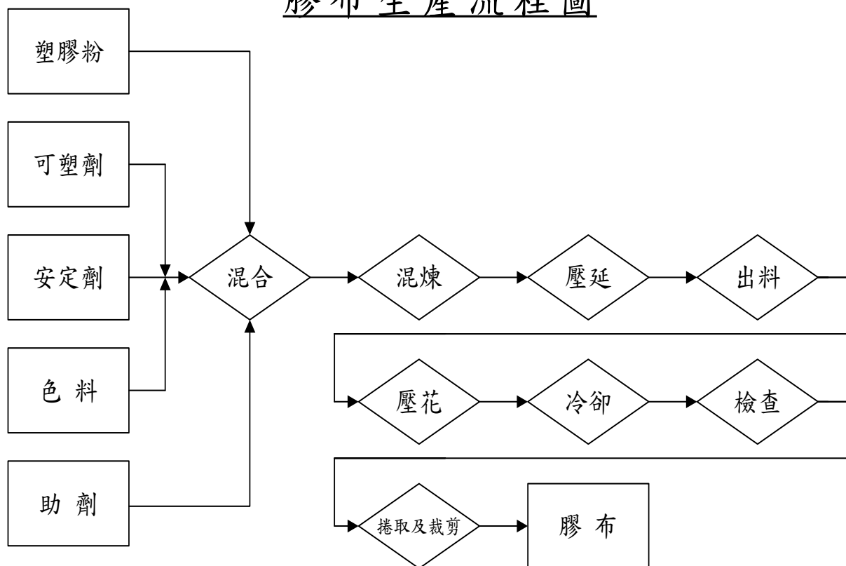
膠布生產流程圖
