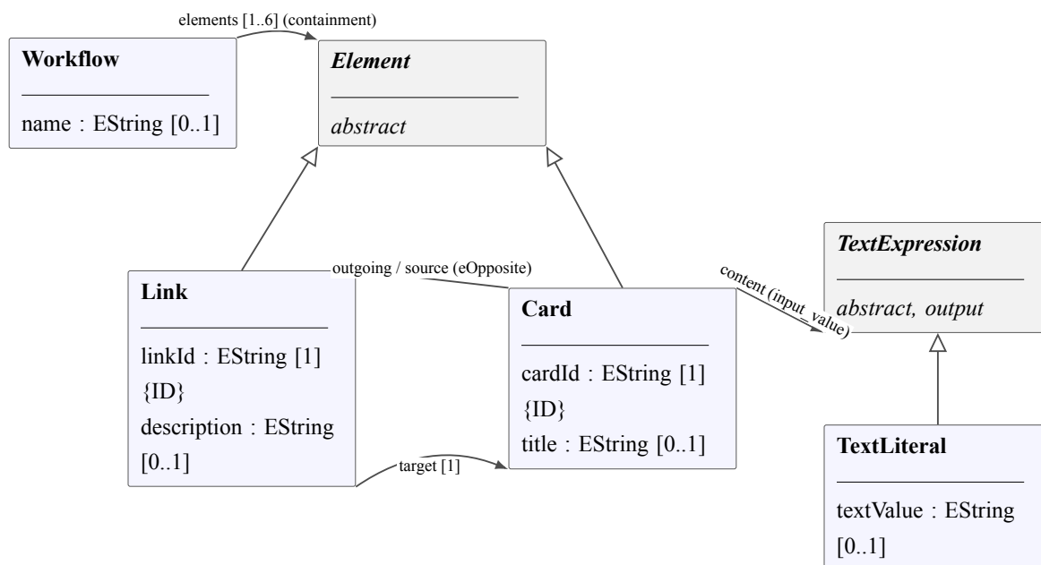
Figura 5.4: Vista parcial del Ecore del ejemplo 03_relations
