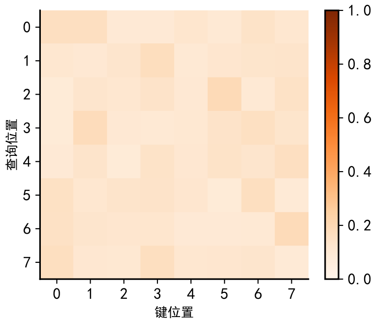
注意力头 3
