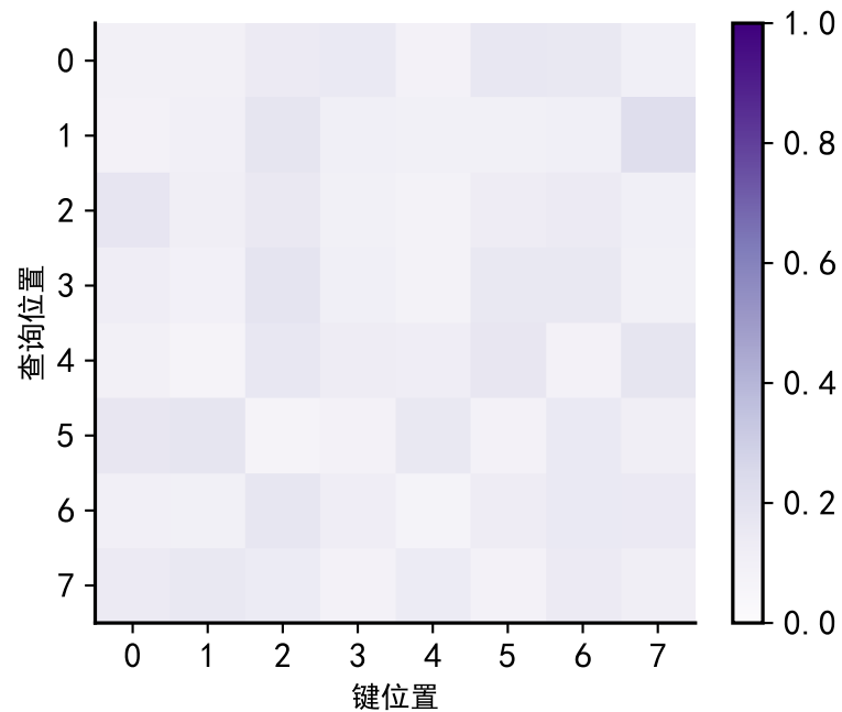
注意力头 4
