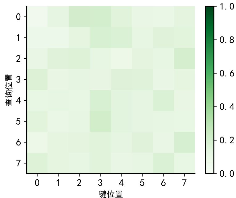
注意力头 2
