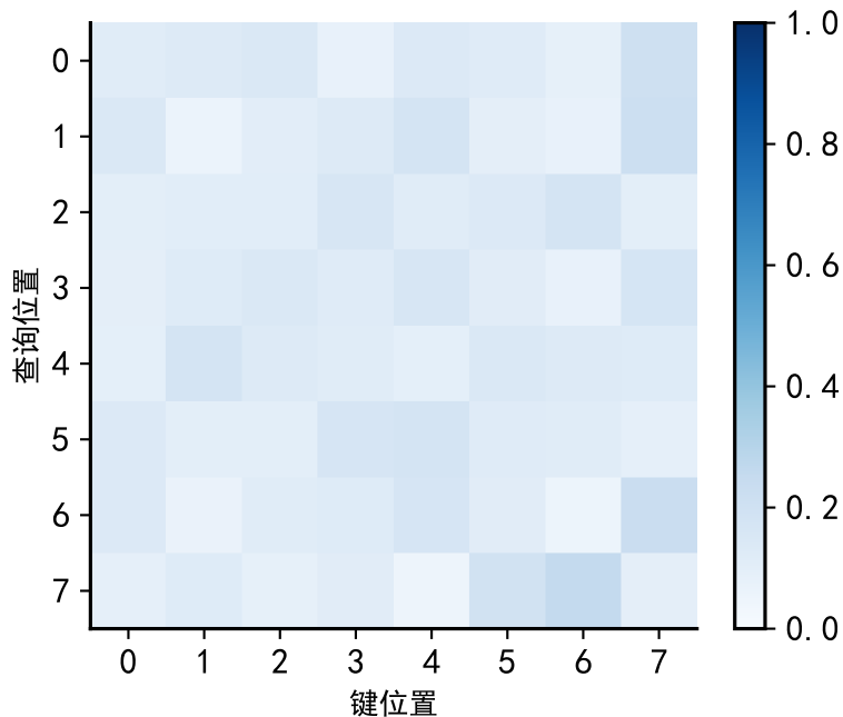
注意力头 1
