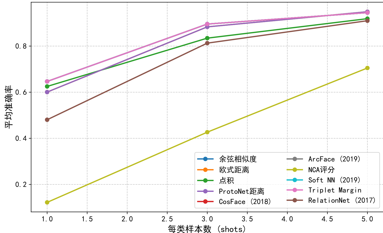
样本数量对不同评分函数的影响
